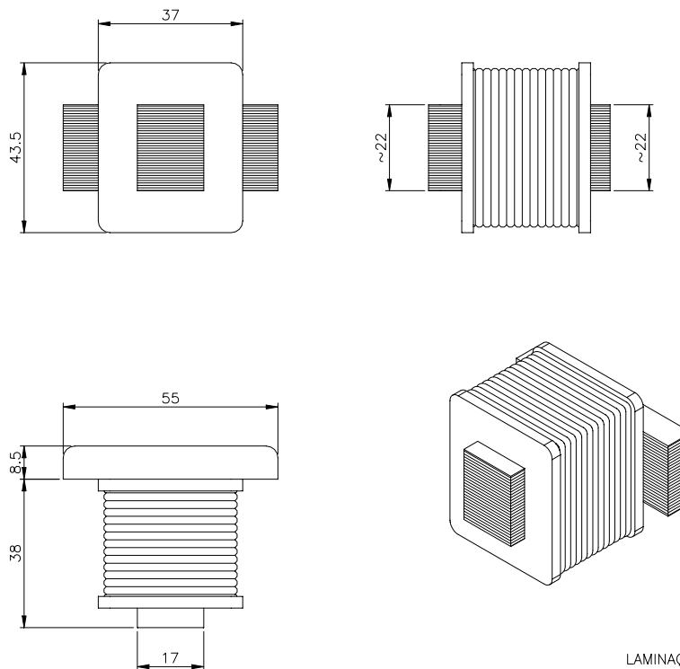
Figura 5 Eletroímã de referência para ensaio da influência da indução magnética CC de origem externa.
