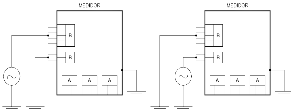
Figura 2b. Ligações a serem feitas para o ensaio de tensão aplicada
